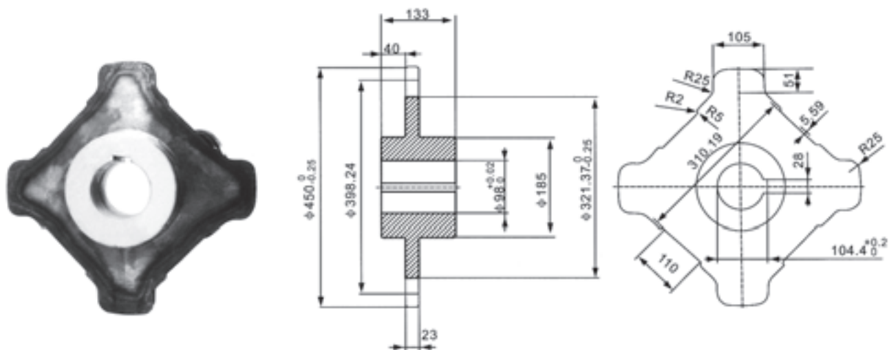
节距 pitch : 152.4 齿数 number or teeth : 4Z 滚子直径 roller diameter : \phi 46
